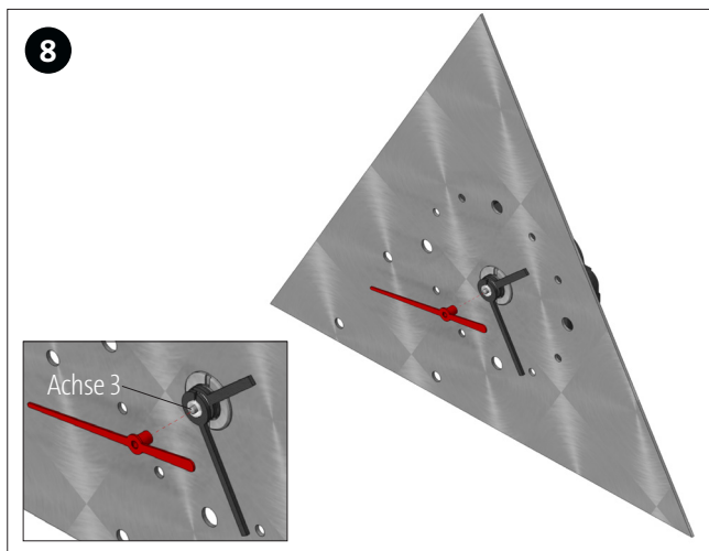
Den Sekundenzeiger auf die Quarzwerkachse (3) aufstecken.
