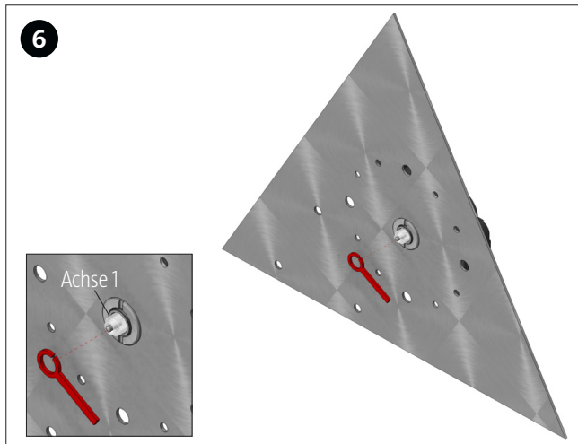
Den Stundenzeiger auf die Quarzwerkachse (1) aufstecken.
