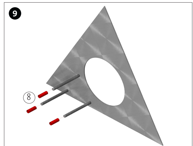
Von der Vorderseite des Teils (1) jeweils eine Messinghülse (8) auf die Schrauben (6) aufstecken.
