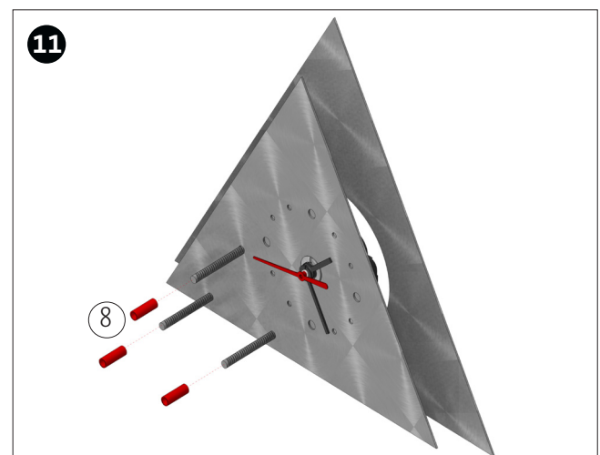
Von der Vorderseite des Teils (2) jeweils eine Messinghülse (8) auf die Schrauben (6) aufstecken.
